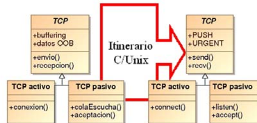
Figura 7: Aplicación de parte del itinerario de C/Unix a los conceptos de Sockets
